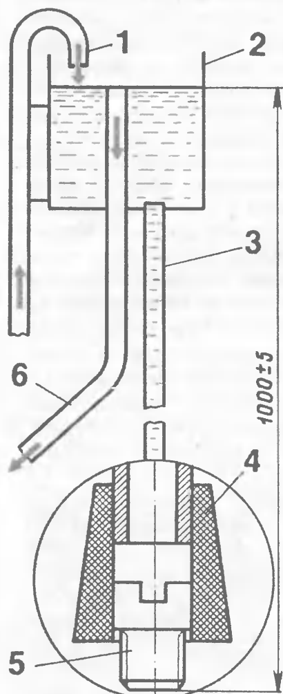
Рис. 1. Схема прибора для определения пропускной способности жиклеров: 1 — шланг для наполнения прибора, присоединяемый к водопроводному крану; 2 — емкость для накопления воды и поддержания постоянной высоты столба жидкости; 3 — трубка для создания столба жидкости над жиклером; 4 — резиновая пробка; 5 — проверяемый жиклер; 6 — шланг для слива избытка воды из емкости.
