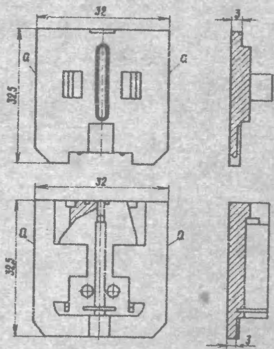
Рис. 1. Корпус карбюратора К-301 (К-302): 1 — направляющая корпуса дросселя; 2 — направляющая щеки дросселя.
