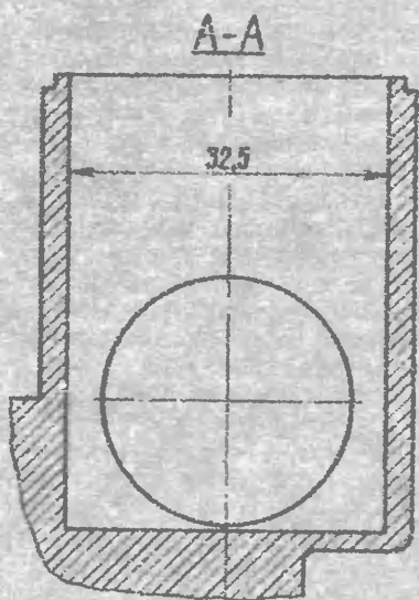
Рис. 2. Корпус (внизу) и щека дросселя карбюратора К-301 (К-302): а — боковые поверхности.
